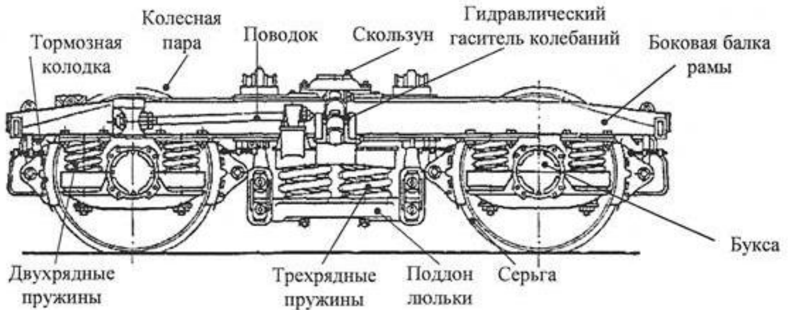
Рис. 10 Тележка КВЗ-ЦНИИ , вид сбоку
