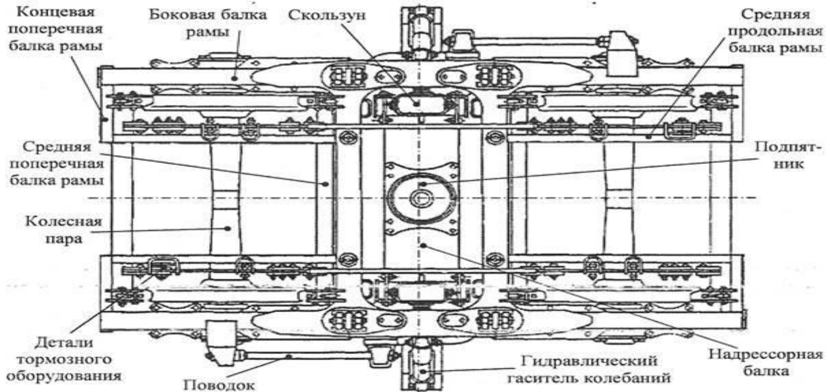
Рис. 9 Тележка КВЗ-ЦНІІ, вид сверху
